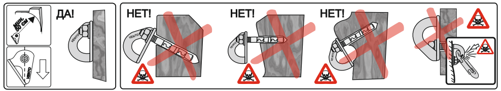
Рис. 6. Положение анкерного устройства и карабина
