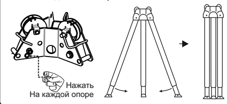
Рис. 5. Регулировка высоты
